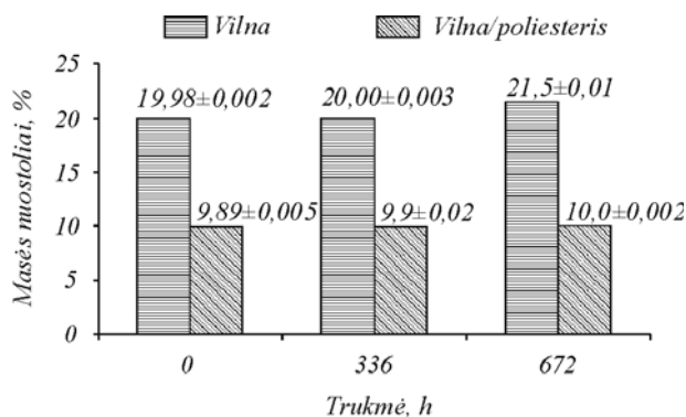
5 pav. Vilnonio ir mišraus pluošto (vilna / poliesteris) audinių, veikiamų natūraliomis sąlygomis, bandinių masės nuostoliai, nustatyti tirpumo NaOH tirpale metodu prieš tai bandinius išplovus distiliuotu vandeniu
