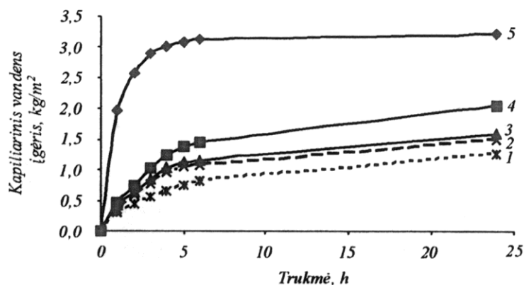
4 pav. Bandomųjų dažų dangų kapiliarinio vandens įgėrio priklausomumas nuo hidrofovizatoriaus bei hidrofovizavimo būdo: 1 – į dažus dedant 1,5 % aminosiloksaninės emulsijos; 2 – 1,5 % silikoninės dervos emulsijos; 3 – 1,5 % aminosiloksaninės emulsijos; 4 – sukietėjusią dangą apdorojant hidrofovizaviniu skysčiu; 5 – nehidrofovizuota danga
