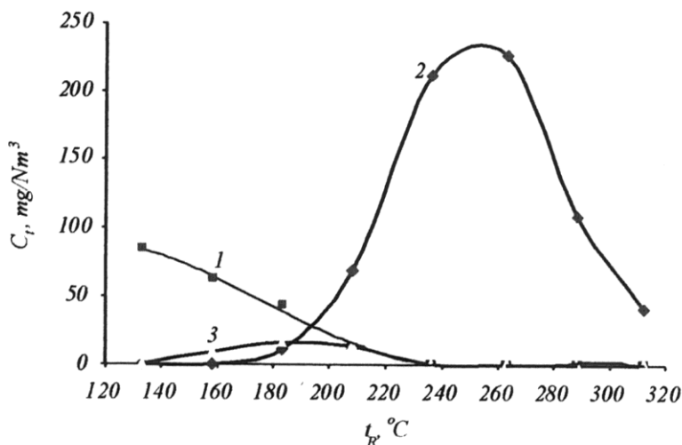
3 pav. Propilacetato katalizinio oksidavimo ant adsorbento-katalizatoriaus CuO / NaX reakcijos produktų srauto sudėties ( C_i ) priklausomumas nuo reaktoriaus temperatūros ( t_R ), \text{mg/Nm}^3 : 1 – 1-propilacetatas; 2 – CO; 3 – 1-propanolis
