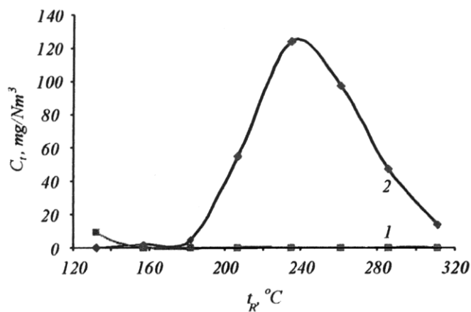
4 pav. Butilacetato katalizinio oksidavimo ant adsorbento-katalizatoriaus CuO / NaX reakcijos produktų srauto sudėties ( C_r ) priklausomumas nuo reaktoriaus temperatūros ( t_R ), mg/Nm 3 : 1 – 1-butilacetatas; 2 – CO
