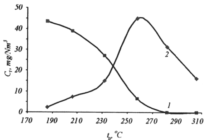
1 pav. Metilacetato katalizinio oksidavimo ant adsorbento-katalizatoriaus CuO / NaX reakcijos produktų srauto sudėties ( C_i ) priklausomumas nuo reaktoriaus temperatūros ( t_R ), \text{mg/Nm}^3 : 1 – metilacetatas; 2 – CO
