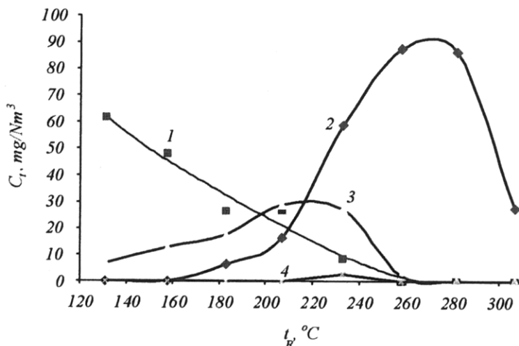
2 pav. Etilacetato katalizinio oksidavimo ant adsorbento-katalizatoriaus CuO / NaX reakcijos produktų srauto sudėties ( C_i ) priklausomumas nuo reaktoriaus temperatūros ( t_R ), \text{mg/Nm}^3 : 1 – etilacetatas; 2 – CO; 3 – etanolis; 4 – dietileteris
